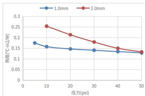
热阻 VS 压力 曲线 (T=1.0mm &amp; 2.0mm)
