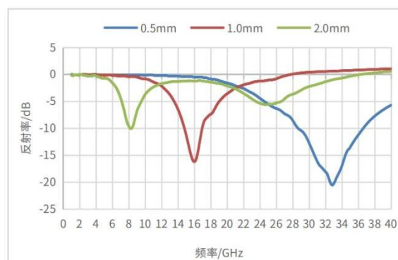
反射率曲线 (T=0.5mm&amp;1.0mm&amp;2.0mm)
