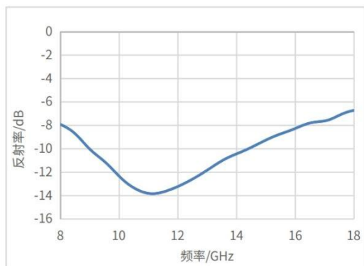
反射率曲线 (T=1.0mm)
