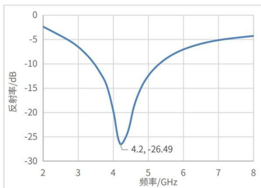
反射率曲线 (T=2.2mm)
