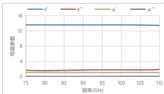
电磁参数 (75~110GHz)
