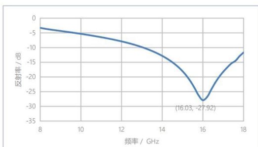
反射率曲线 (T=1.0mm)
