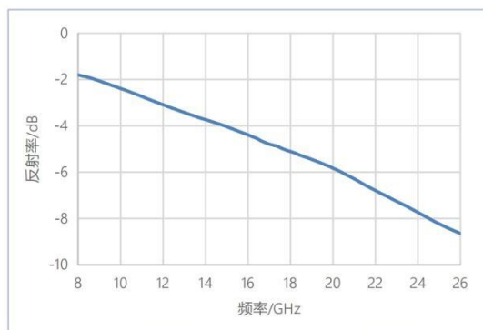
反射率曲线 (T=0.5mm)
