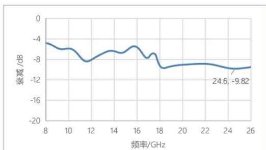
自由场透射曲线 (2~18GHz)
