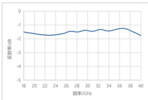
反射率曲线 (T=0.3mm)
