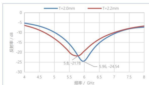
反射率曲线 (T=2& 2.2mm)
