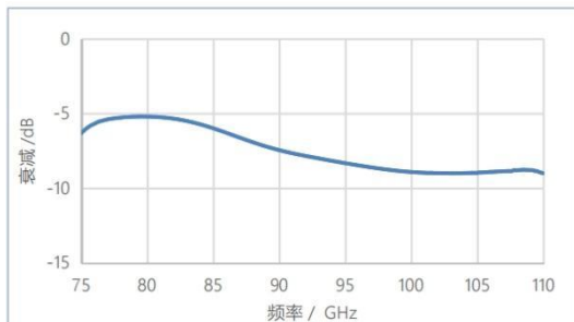
自由场透射曲线 (75~110GHz)
