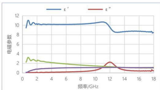
电磁参数 (2~18GHz)
